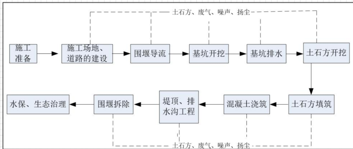
图 2-4 堤防、固床河堰施工工艺图
