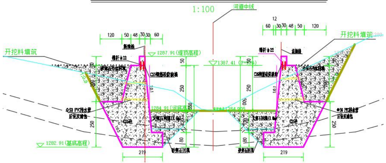
图 2-4 本项目河堤 2 典型断面堤防剖面图
