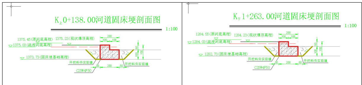
固床坝设计剖面图
